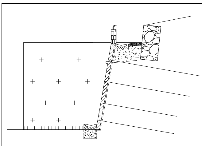
Řez hřebíkovým svahem
