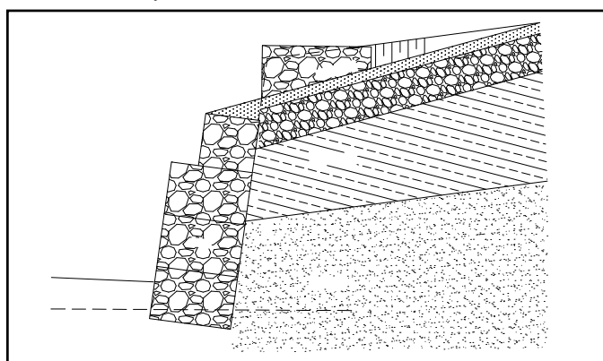
Řez gabiony
