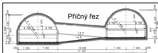
Vzorový příčný řez
