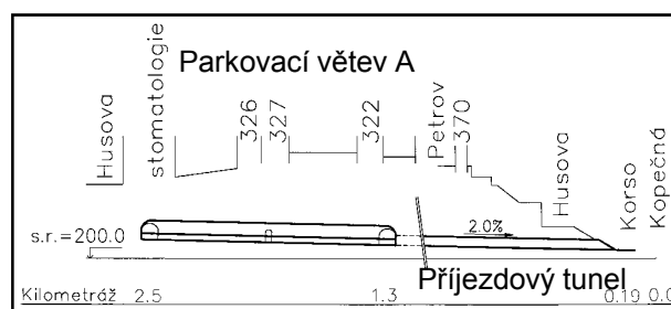
Podélný řez
