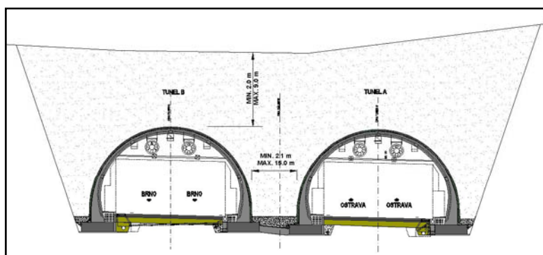
Profil hloubené části tunelu Klimkovice
