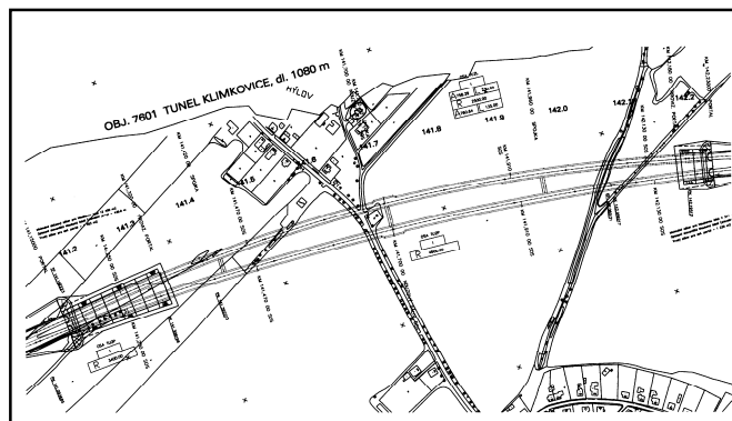
Situace tunelu Klimkovice
