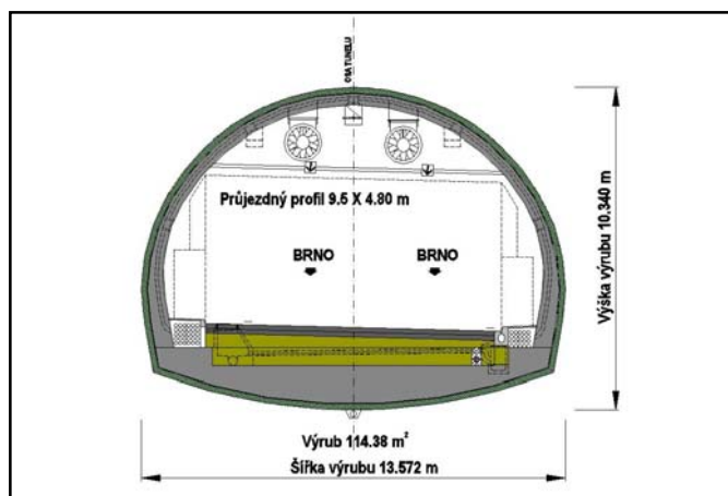
Profil ražené části tunelu Klimkovice
