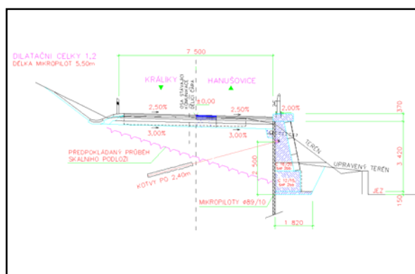
Vzorový příčný řez sanovanou zdí
