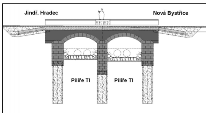
Podélný řez mostem
